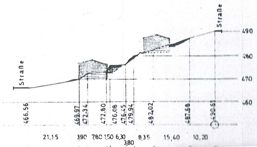
Schnitt B-B
